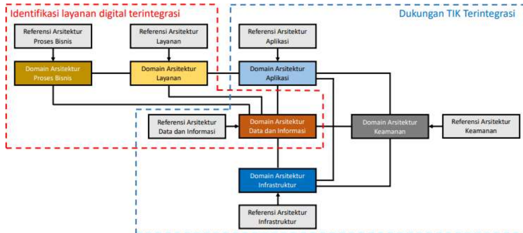
Gambar 7. Keterkaitan antar Referensi Arsitektur SPBE
